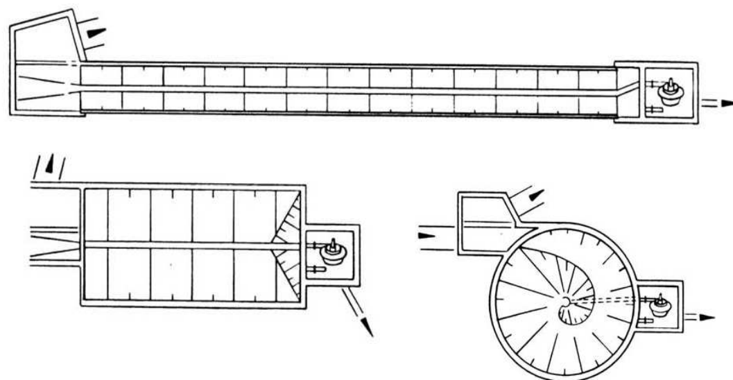
Depósitos de retención en línea
